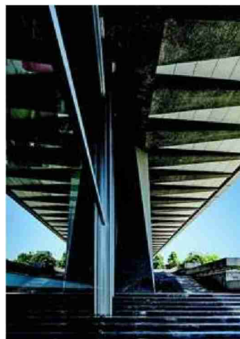
La structure portante du bâtiment de l'OMS à Genève.
